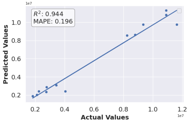
Fig. 3. Actual vs. predicted values for Gradient Boosting model
