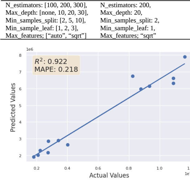
Fig. 5. Actual vs. predicted values for random forest model
